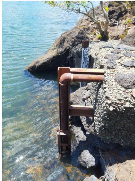
Station limnimétrique de la Rivière de Lacs. Sonde partiellement hors d'eau (18/12/2019)
